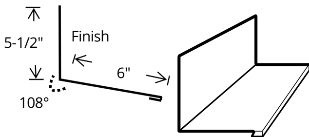
Endwall
