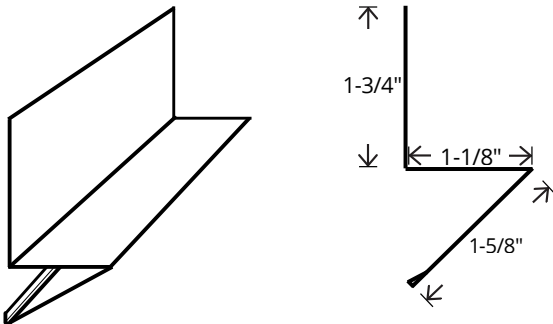
Starter/Box
