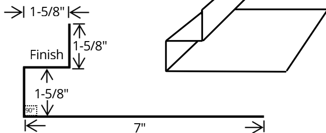
7" Door Jamb Box
